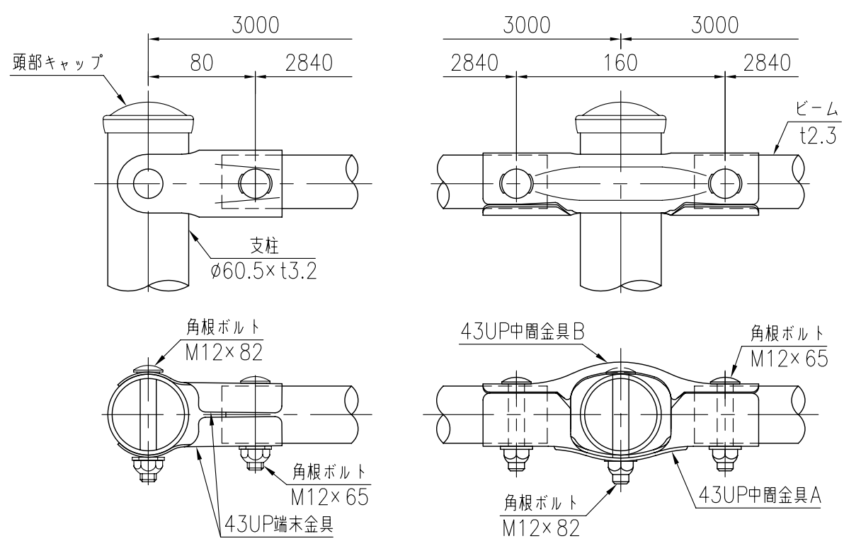
取付部詳細図 (1/4)
