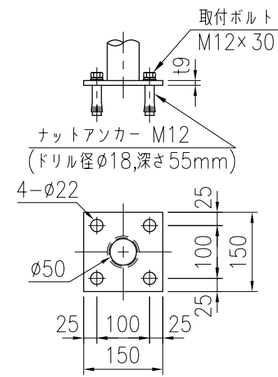
ベースプレート詳細図 (1/10)
