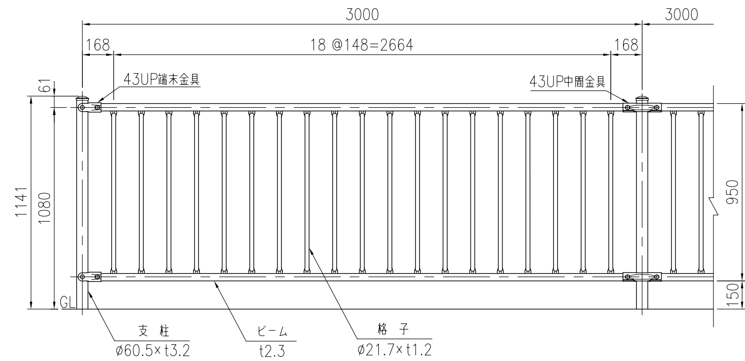
設置図 (1/20)
