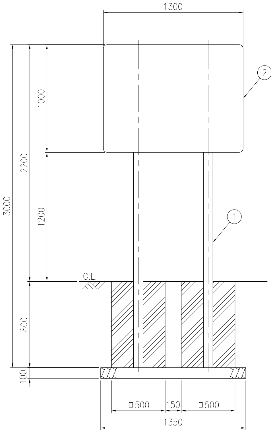
設置図 S=1/20
