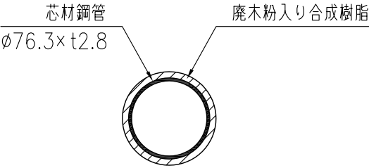
支柱断面詳細図 S=1/5
