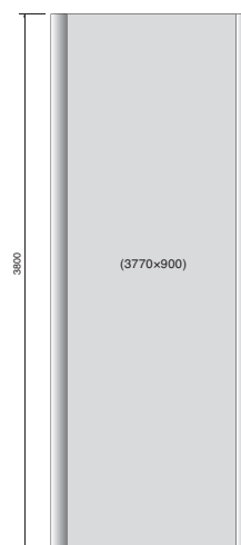
SUS-LM3809-S(W)
