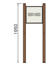
SOW-NAS0606-1S(W)
