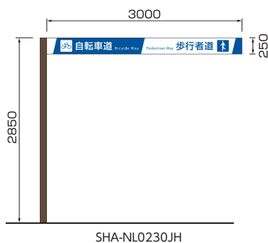
逆L型3000タイプ
