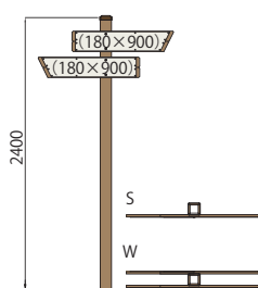
TW-YH0209-2SZ TW-YH0209-2WZ
