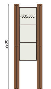
SOW-NAB0606-3S(W)
