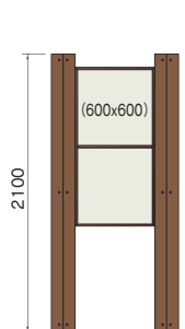
SOW-NAB0606-2S(W)
