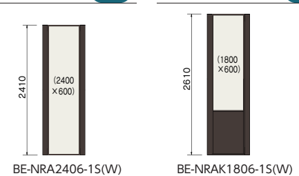
全面パネルタイプ/大型・下部パネルタイプ
