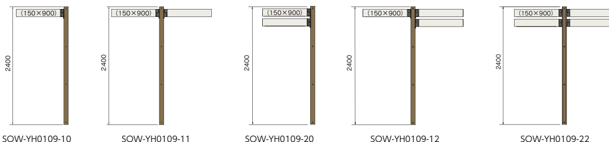
SOW-YH0109-10
