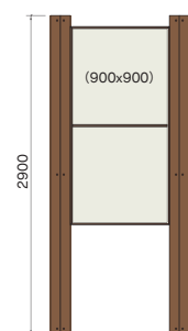
SOW-NAB0909-2S(W)
