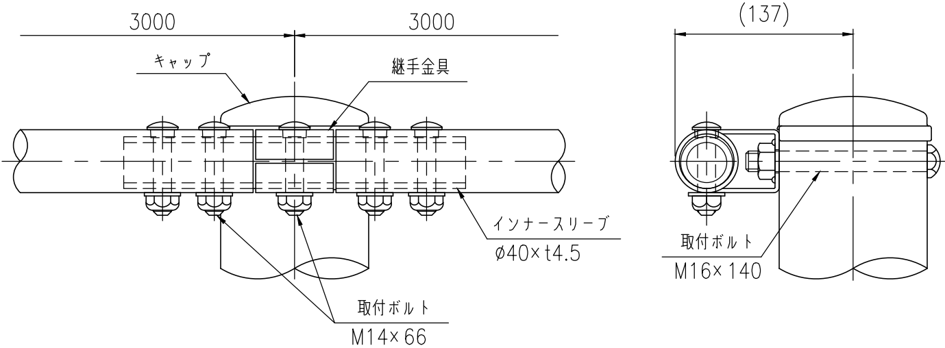
継手部詳細図 (1/4)
