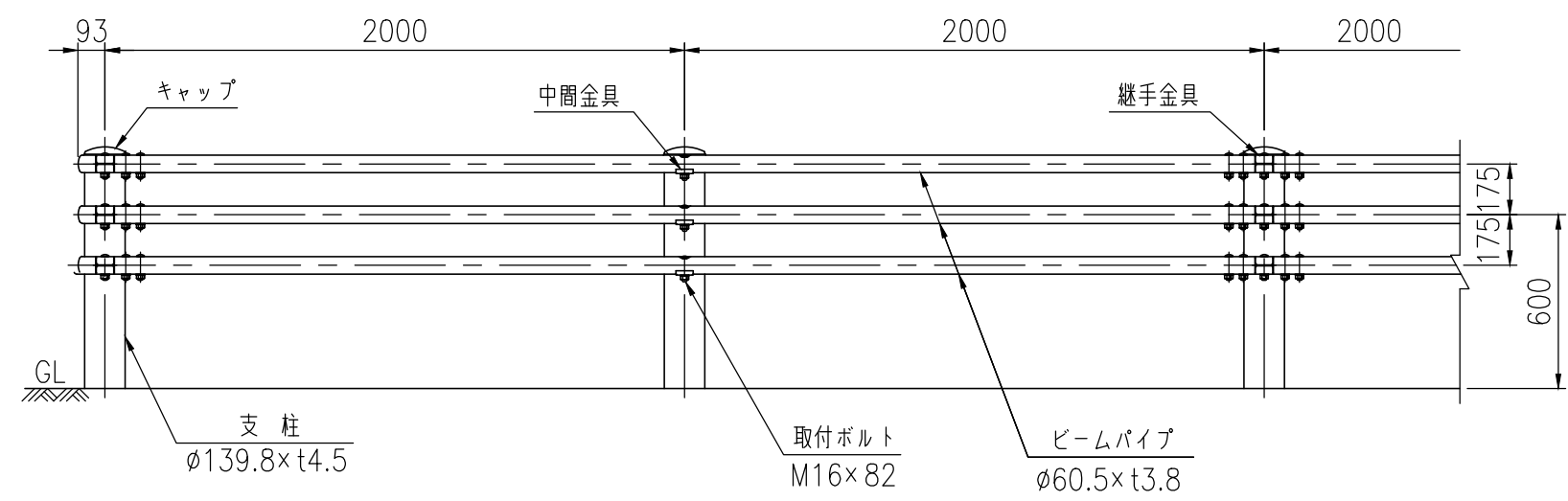
設置図 (1/25)
