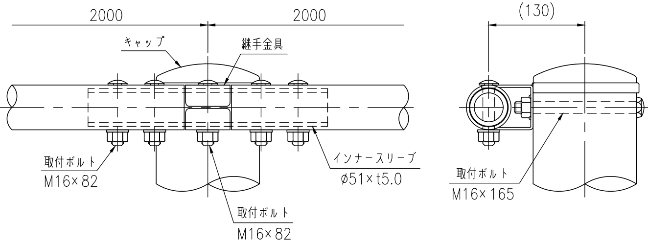
継手部詳細図 (1/5)
