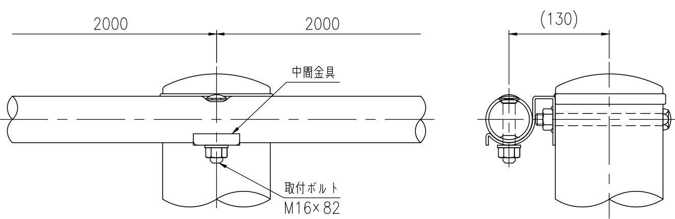
中間部詳細図 (1/5)
