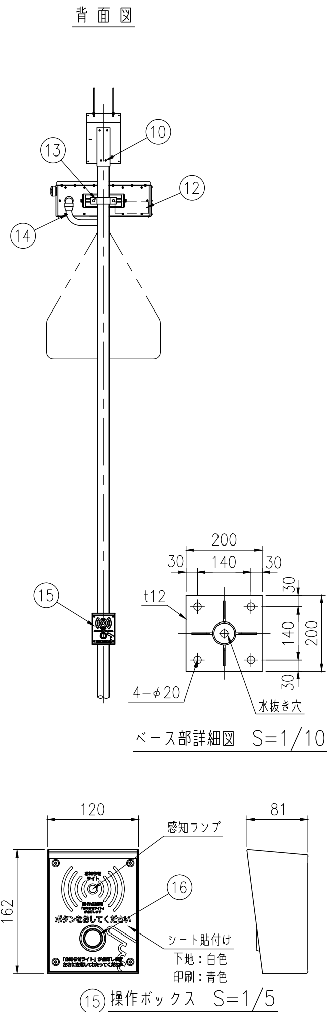
横断者注意喚起灯 ゆずるくん YZR-PB-A-H
