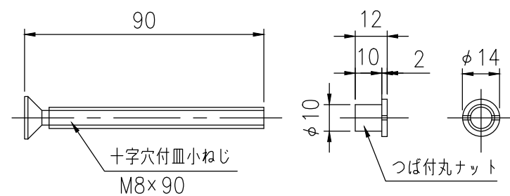
⑥ ボルト・ナット詳細図 S=1/2
