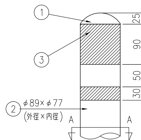
本体上端部 S=1/5
