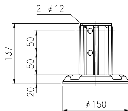
④ ベースプレート詳細図 S=1/5
