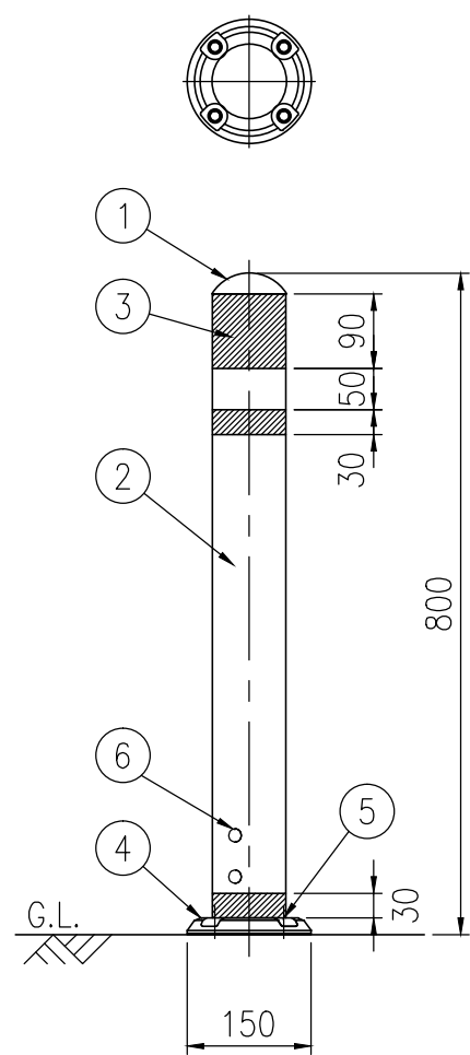
設置図 S=1/10
