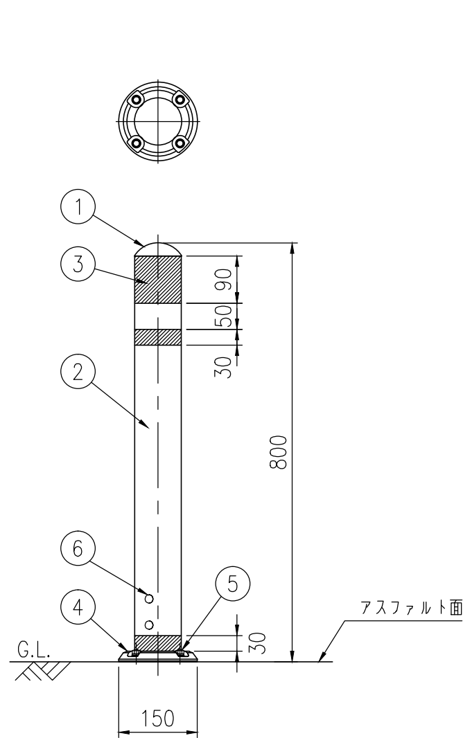
設置図 S=1/10
