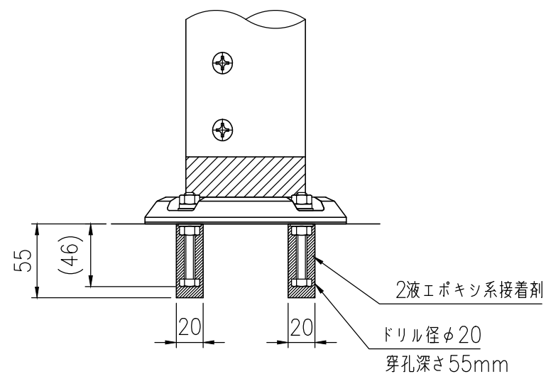
設置図(詳細) S=1/4
