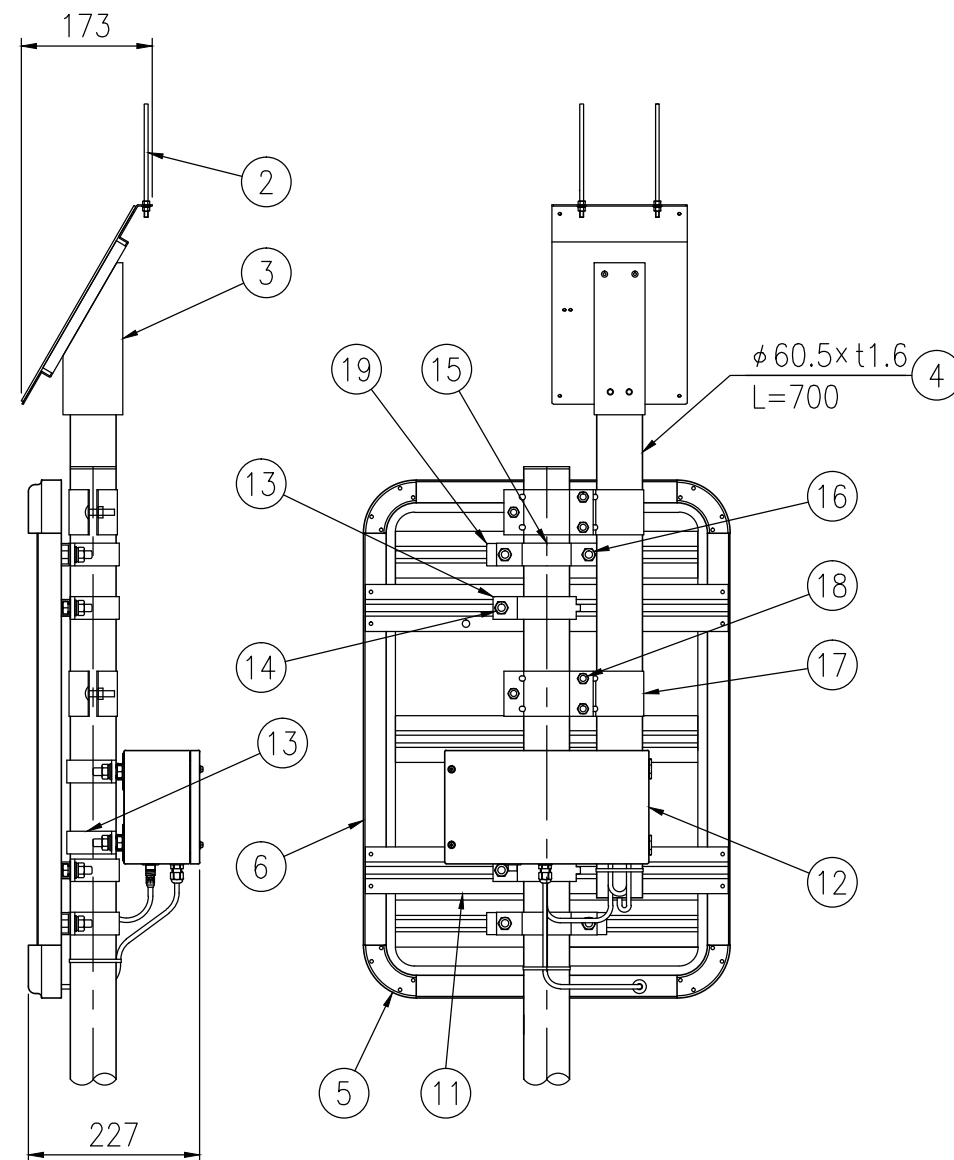
設置図 S=1/10
