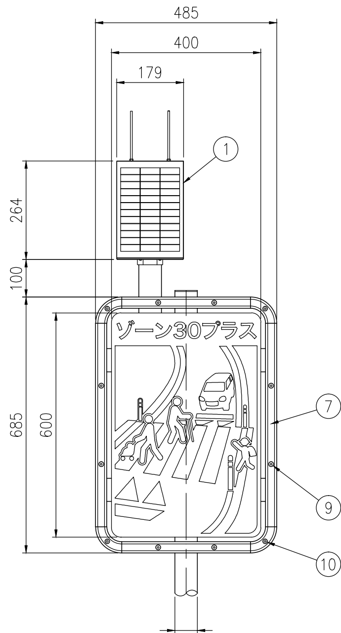
設置図 S=1/10
