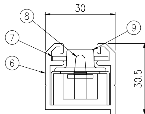
発光体取付詳細図 S=1/1
