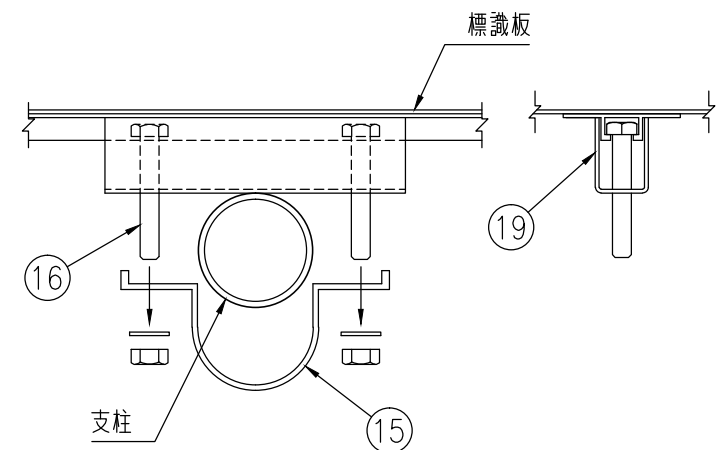
標識板取付部
