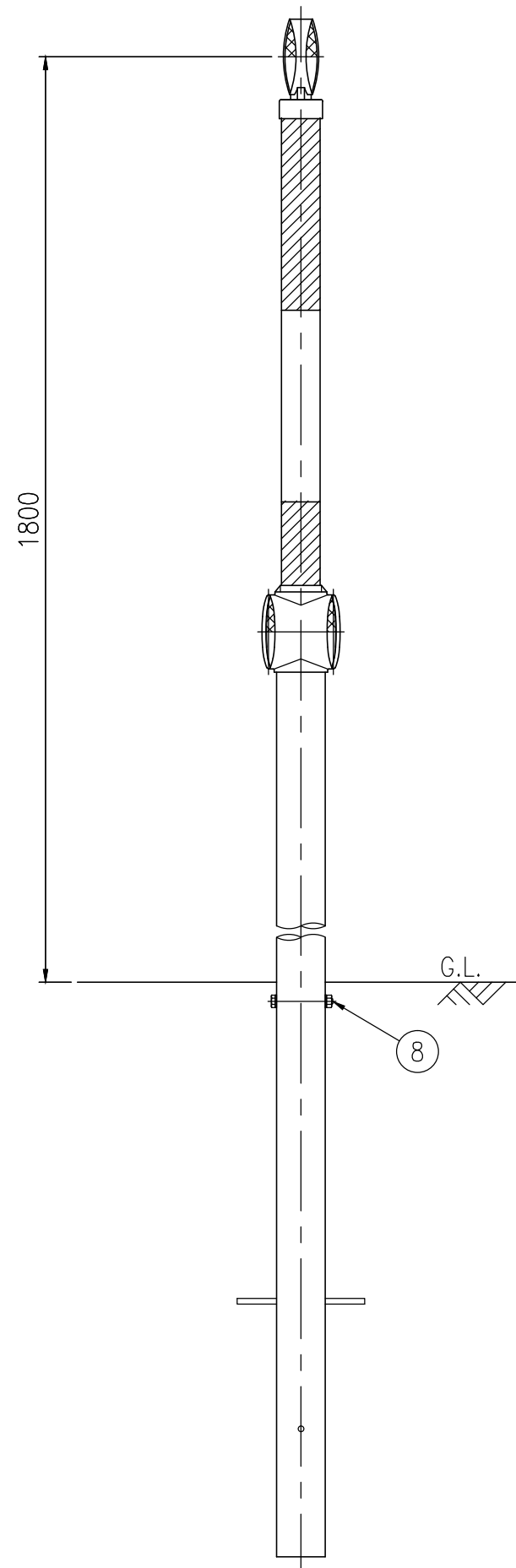
設置図 S=1/10
