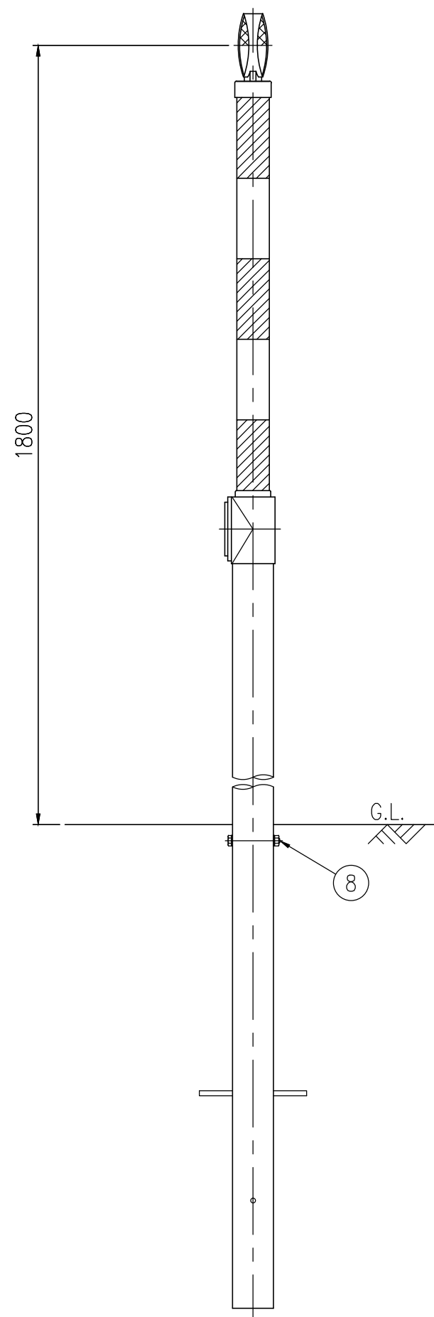
設置図 S=1/10
