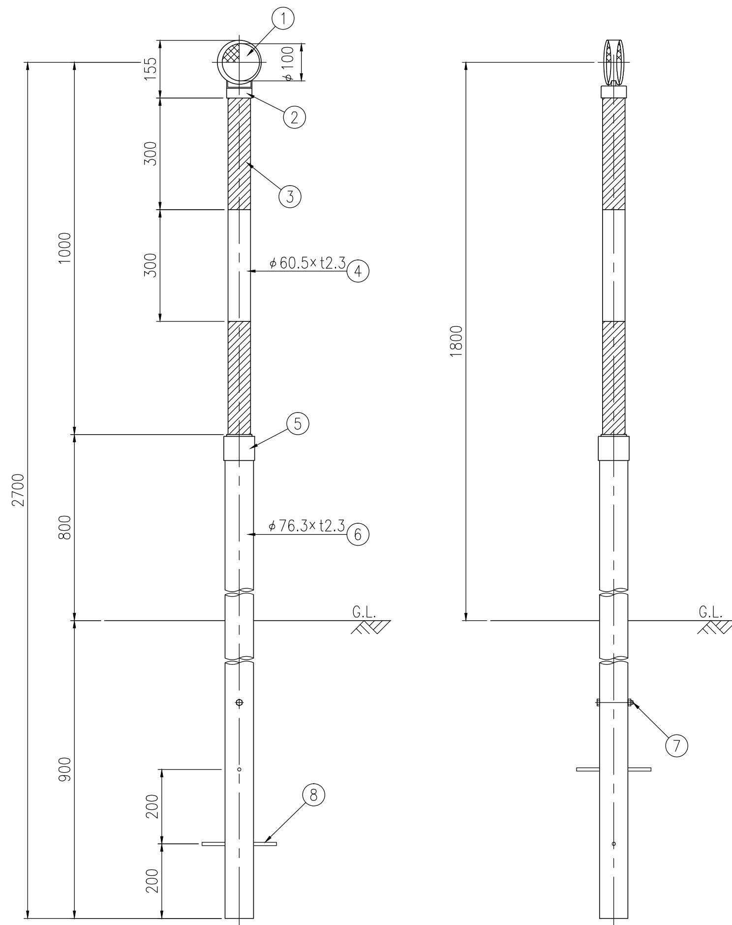
設置図 S=1/10
