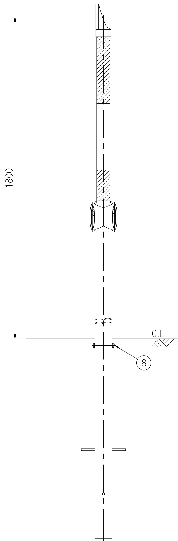
設置図 S=1/10
