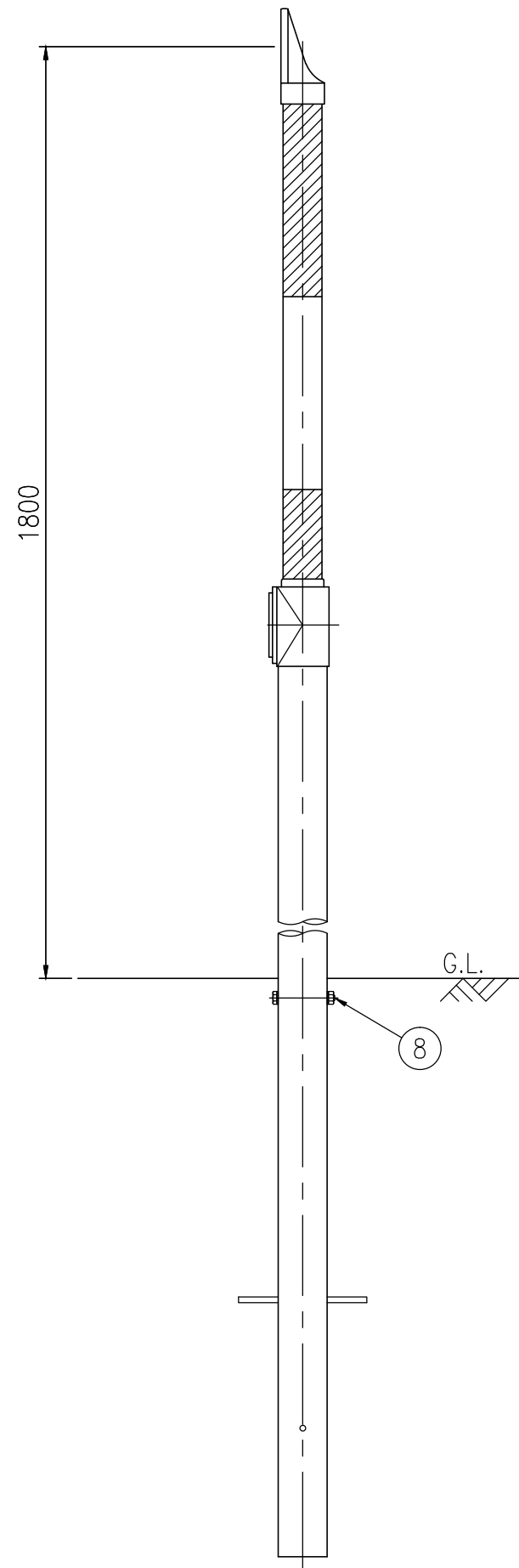
設置図 S=1/10
