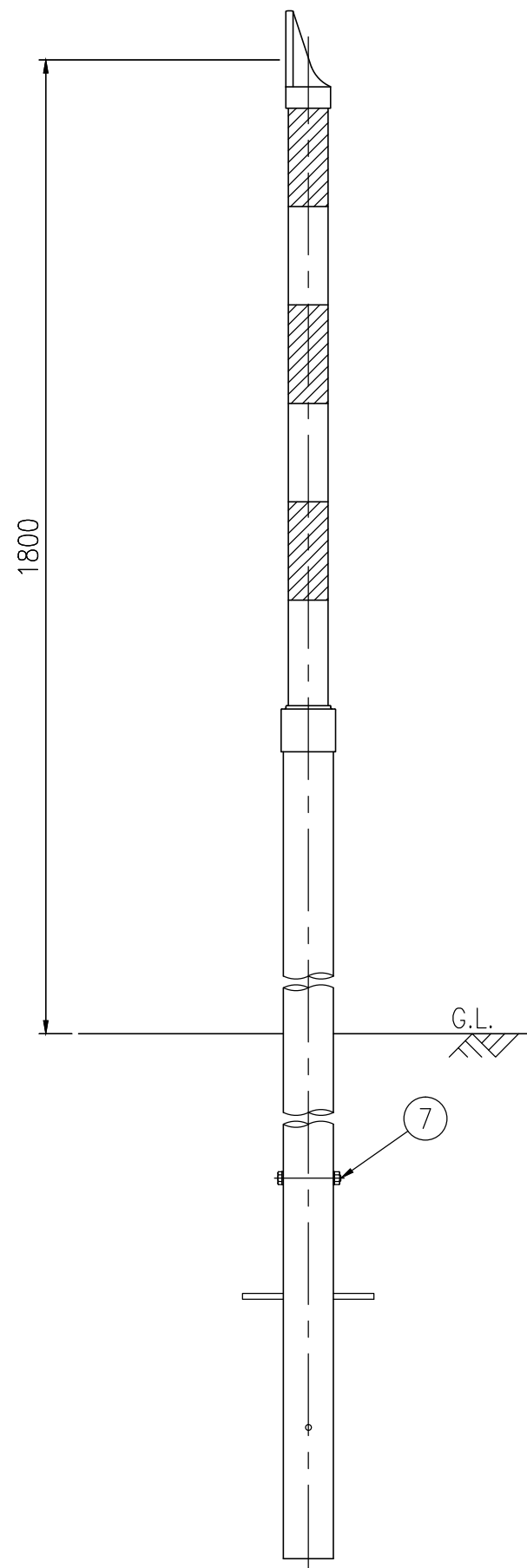
設置図 S=1/10
