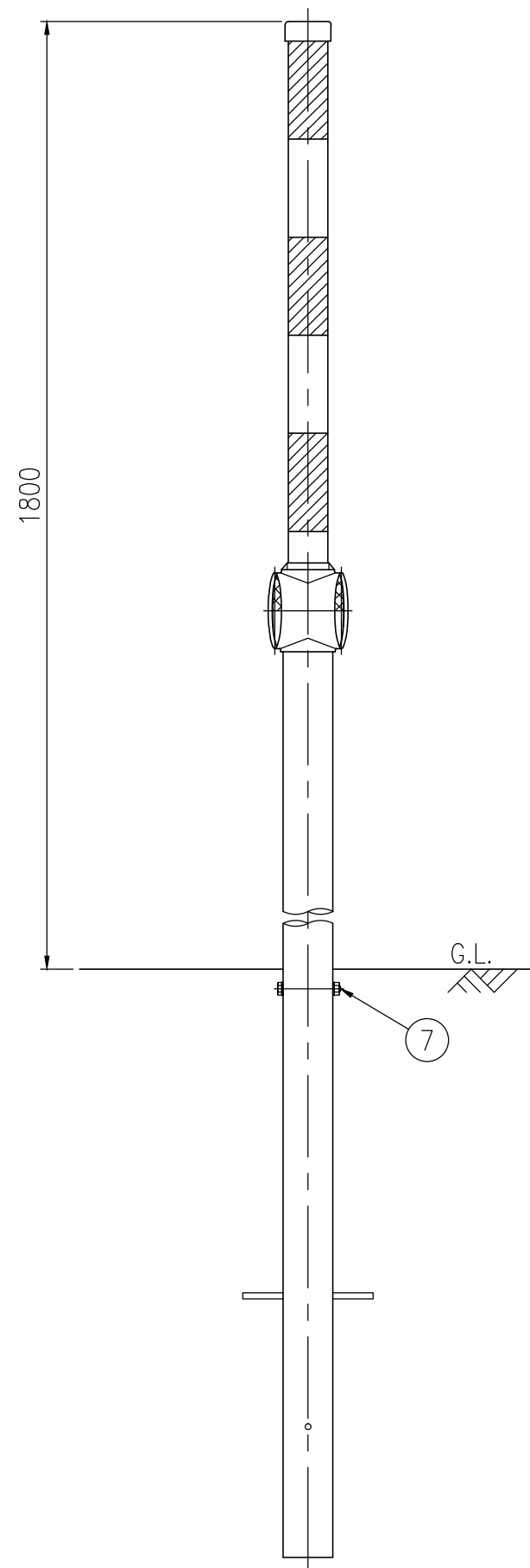
設置図 S=1/10
