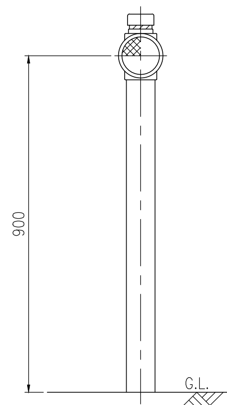
収納時 S=1/10
