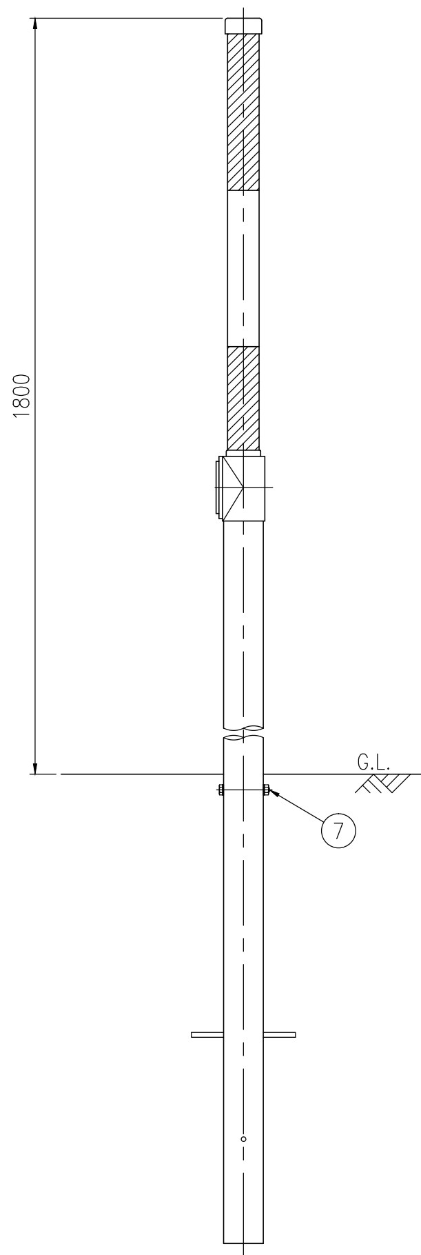
設置図 S=1/10
