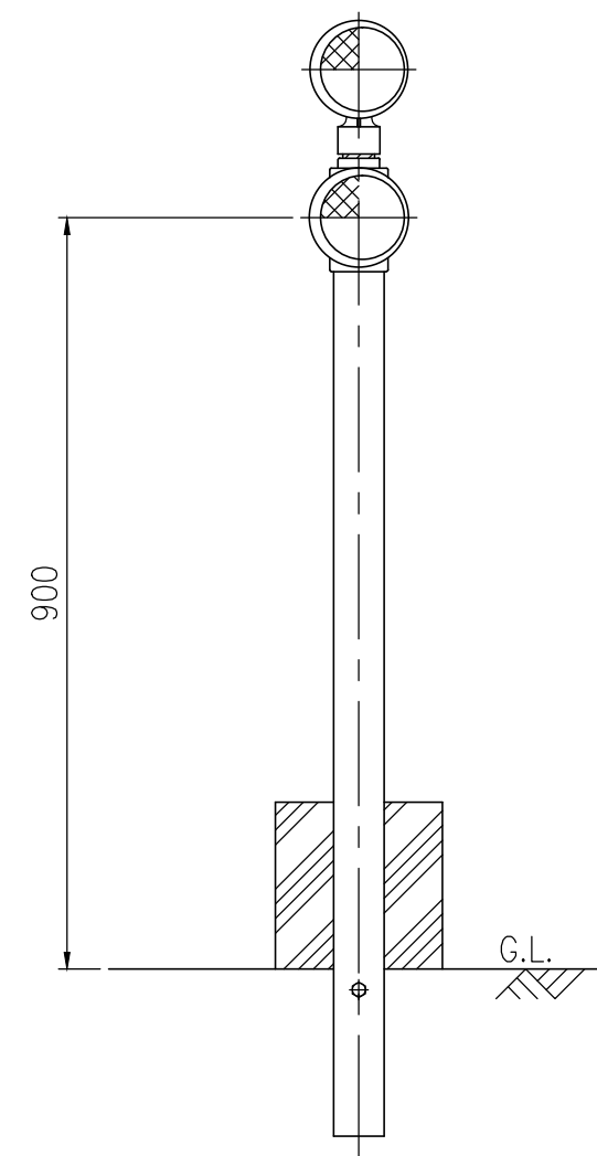
収納時 S=1/10
