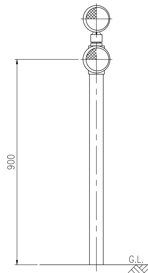
収納時 S=1/10
