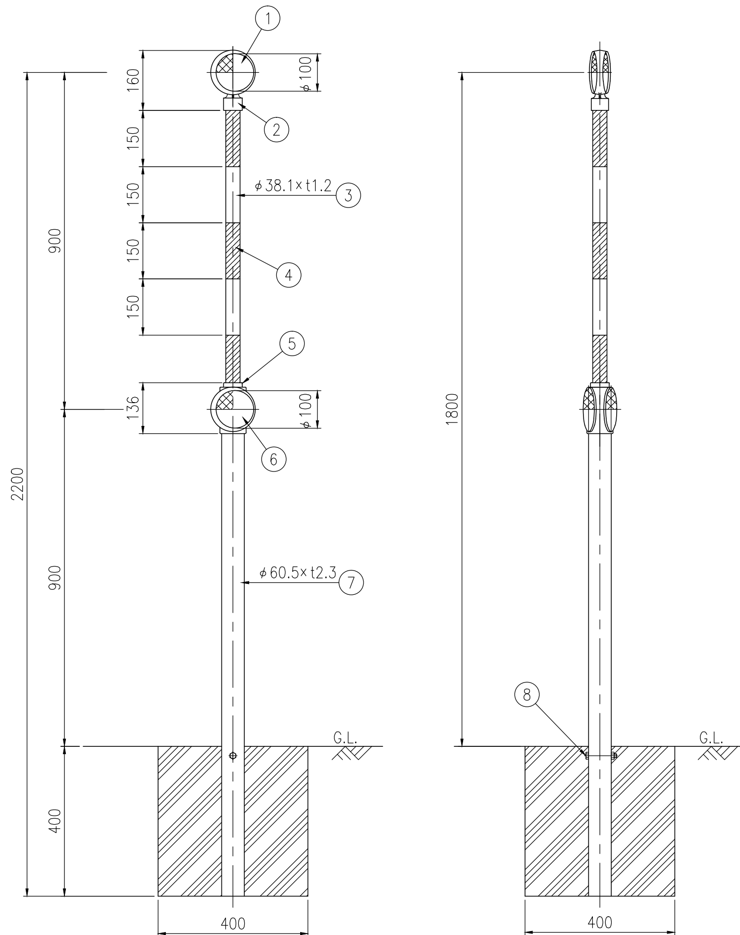
設置図 S=1/10
