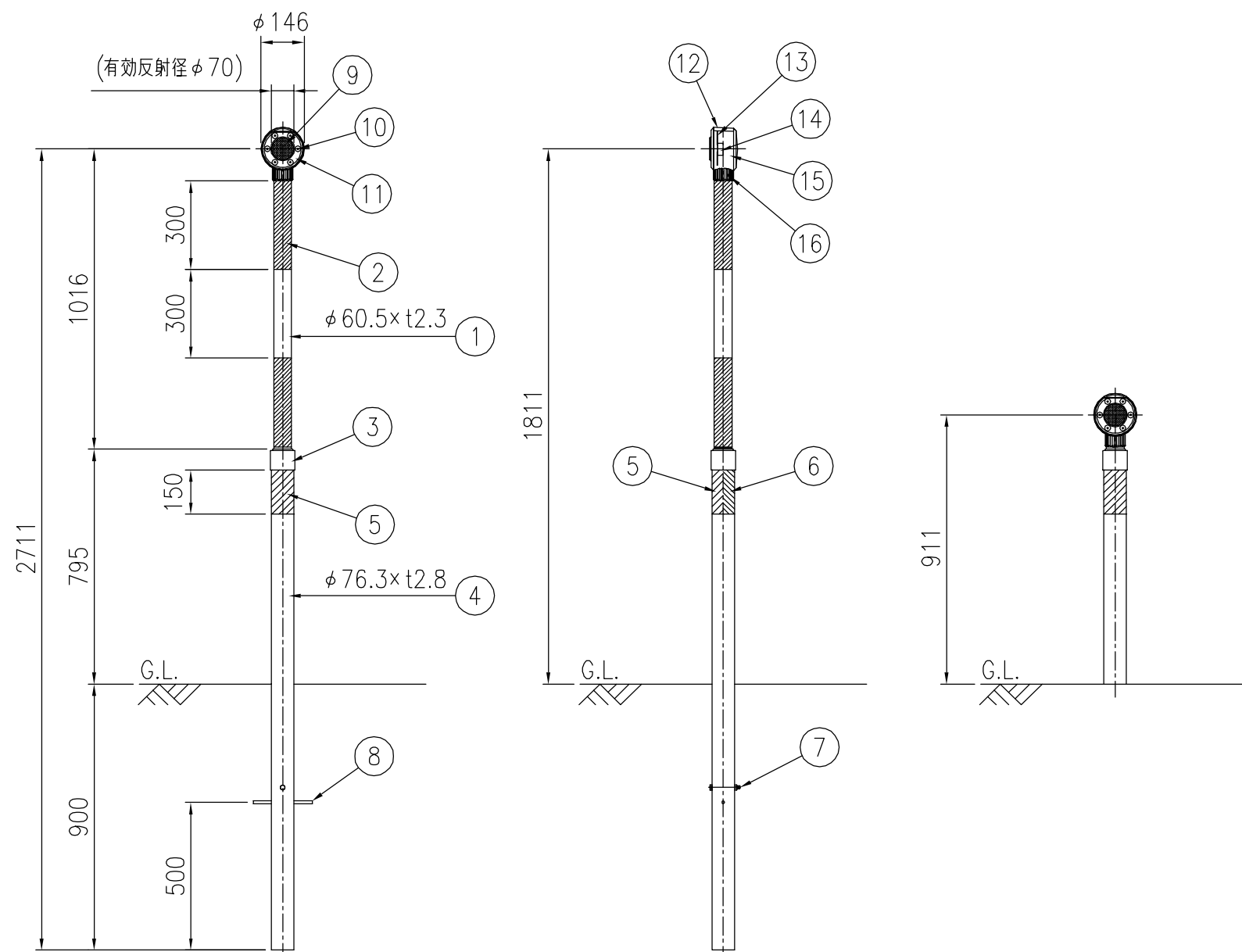
設置図 S=1/20
