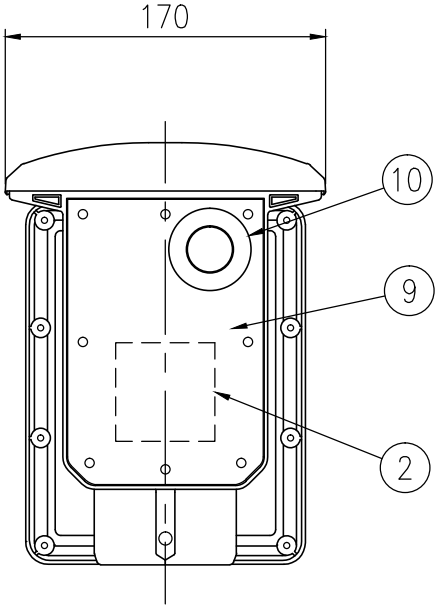
背面図
