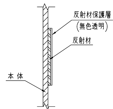
B部断面図
