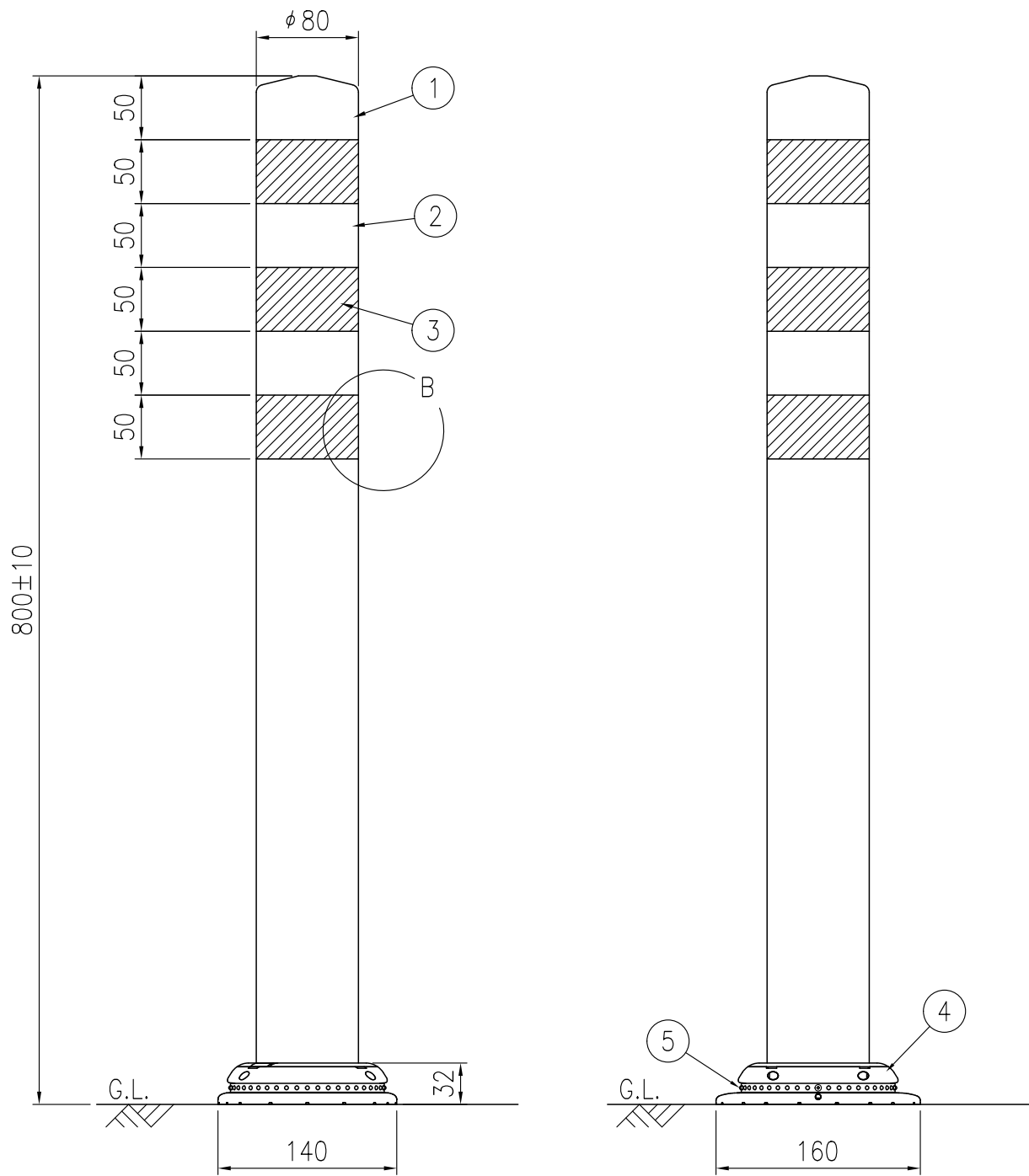
設置図 S=1/5
