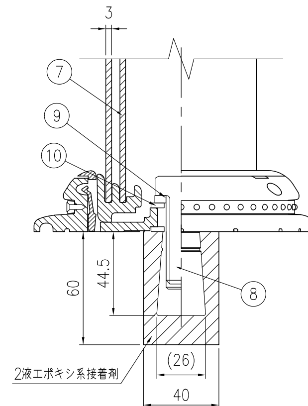
A-A半断面図 S=1/2
