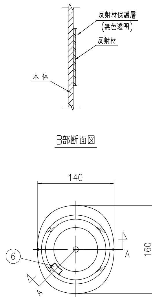
平面図 S=1/4
