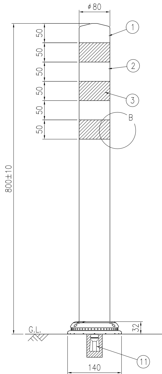
設置図 S=1/5
