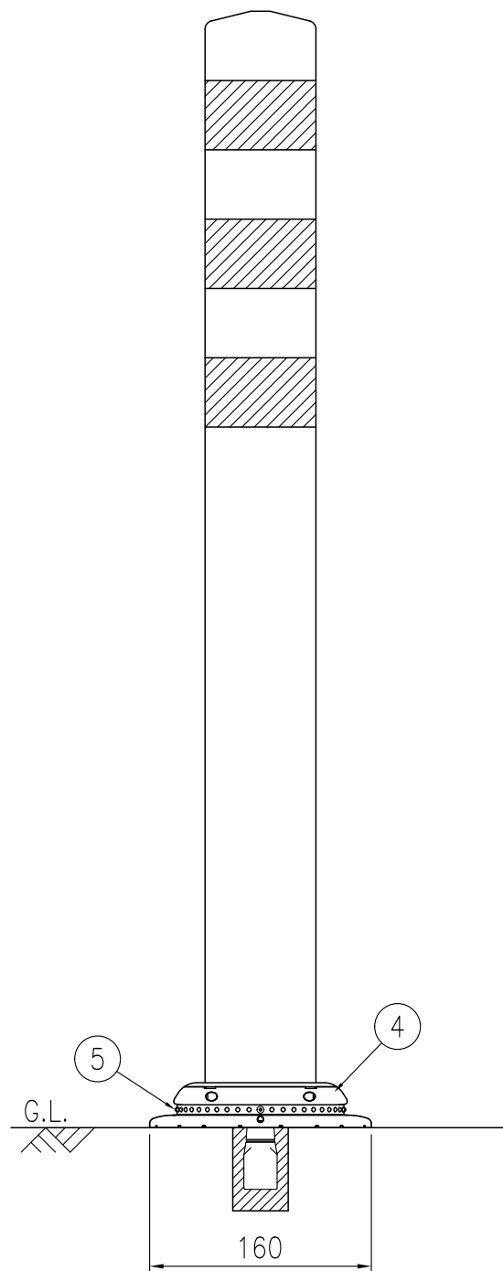
設置図 S=1/5
