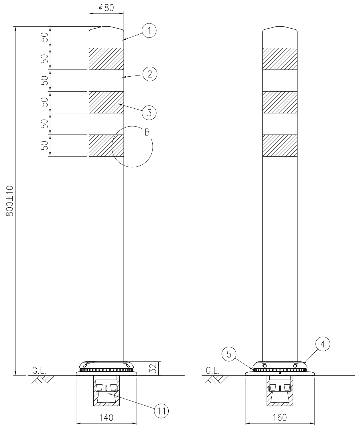
設置図 S=1/5
