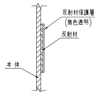
B部断面図
