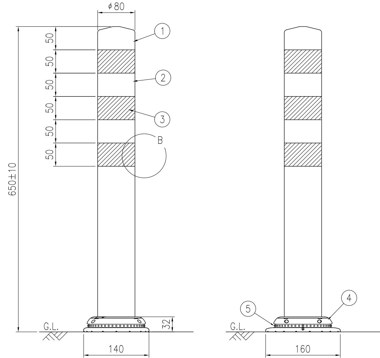
設置図 S=1/5
