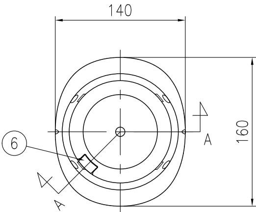
平面図 S=1/4
