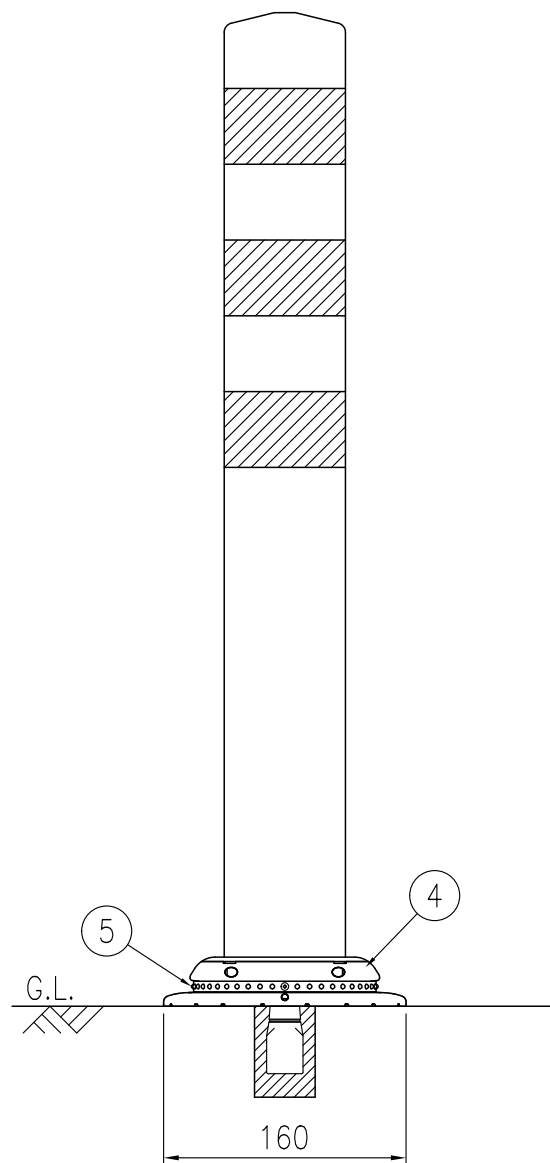
設置図 S=1/5
