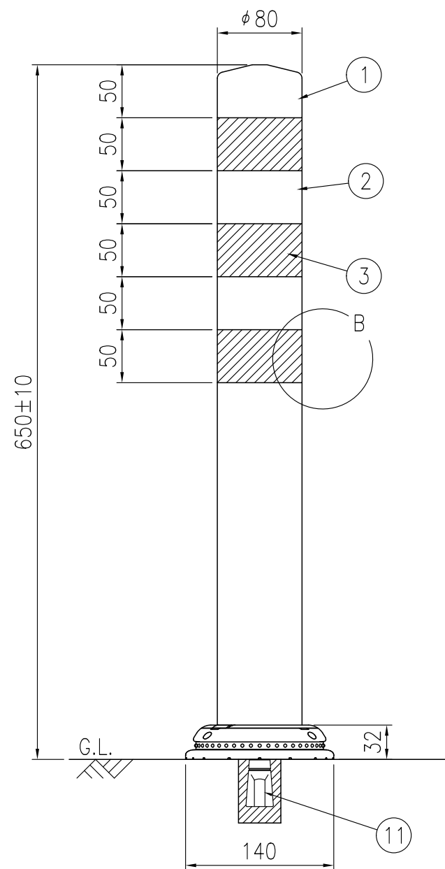
設置図 S=1/5
