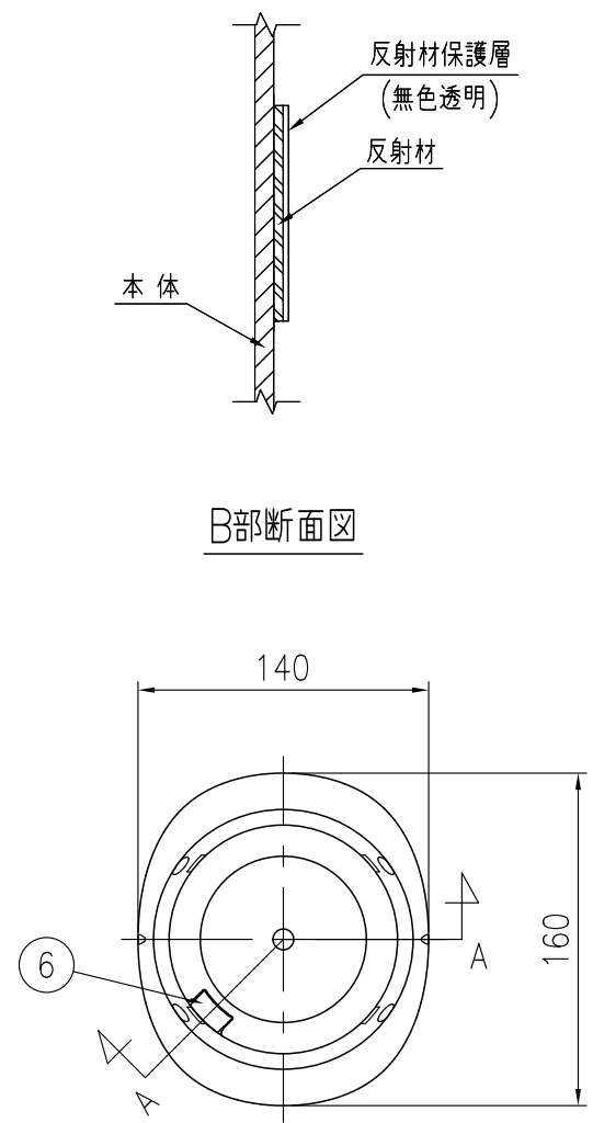
平面図 S=1/4
