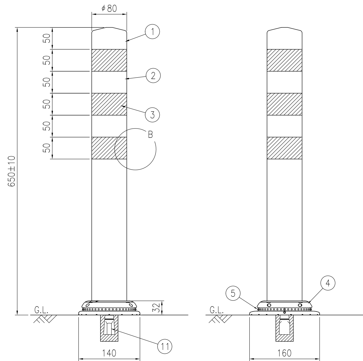
設置図 S=1/5
