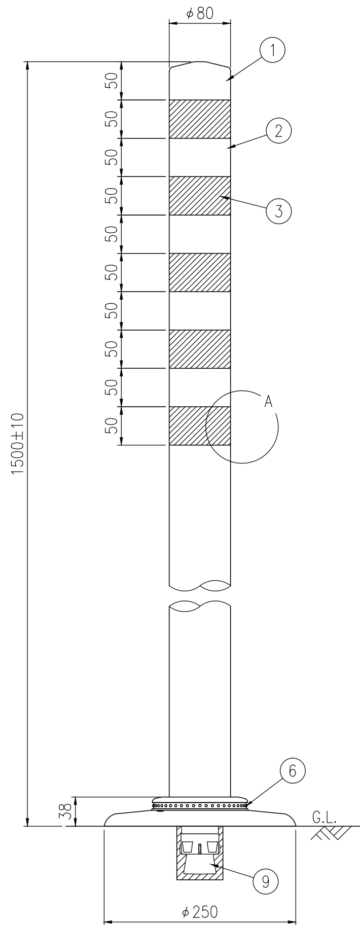
設置図 S=1/5
