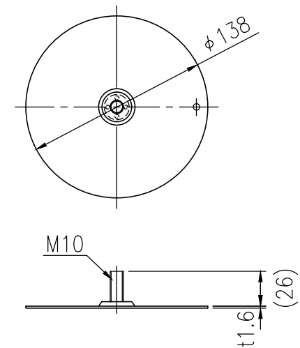
⑧ スチールスペーサー詳細図 S=1/4
