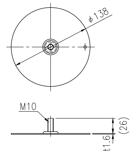
⑦ スチールスペーサー 詳細図 S=1/4
