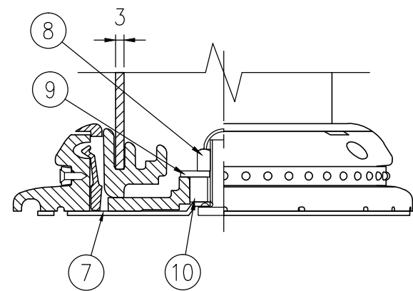
A-A半断面図 S=1/2
