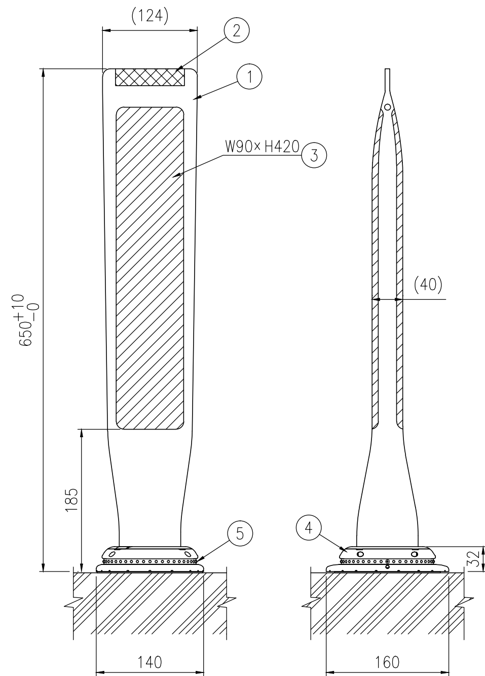
設置図 S=1/5
