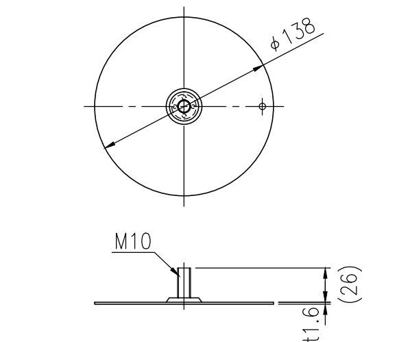
⑦ スチールスペーサー 詳細図 S=1/4
