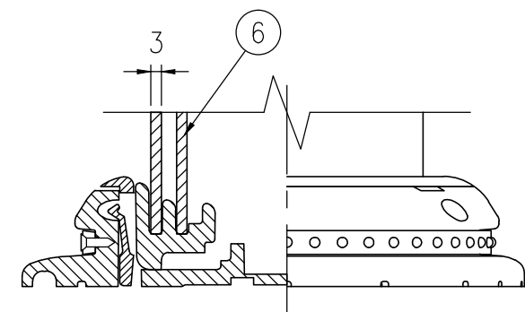
A-A半断面図 S=1/2
