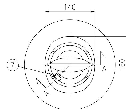
平面図 S=1/5
