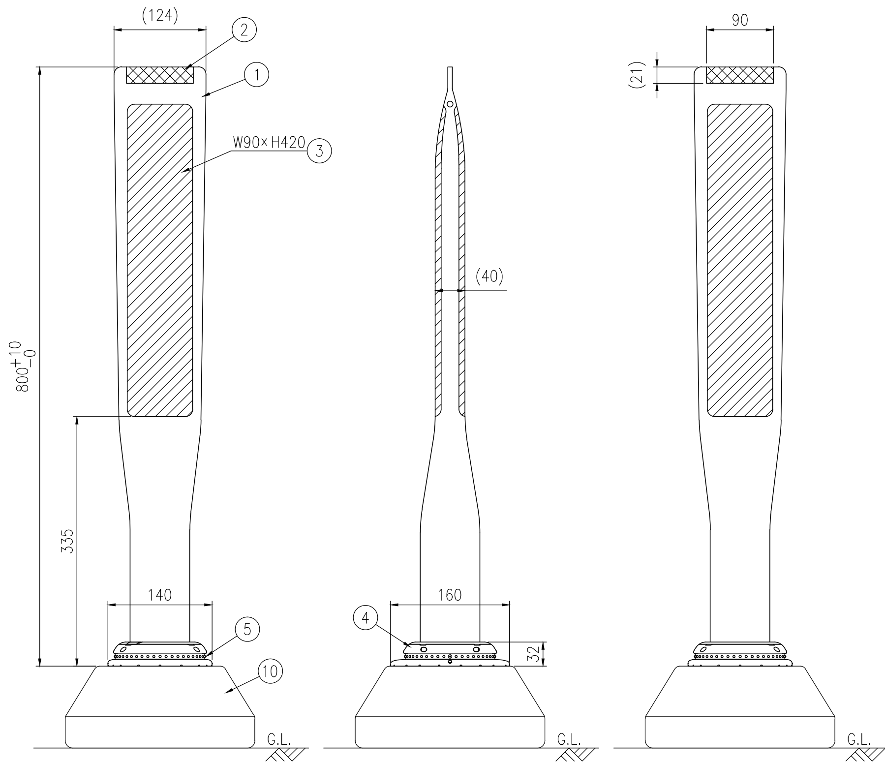
設置図 S=1/5
