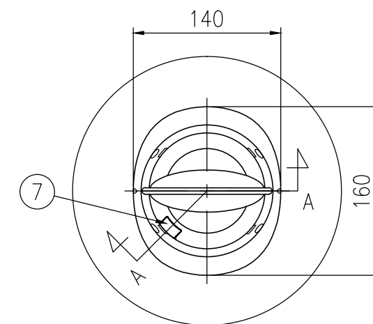
平面図 S=1/5
