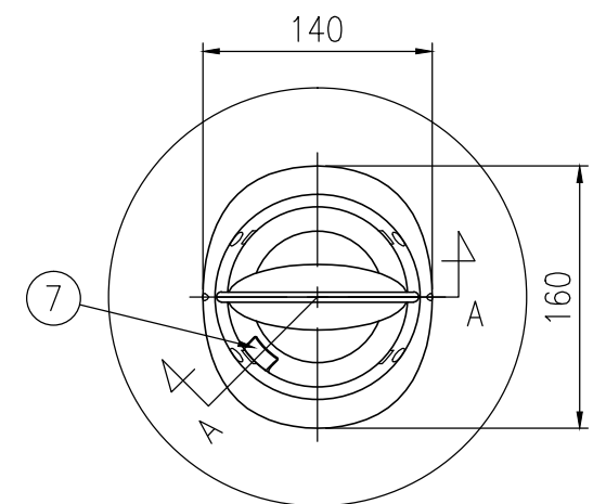
平面図 S=1/5
