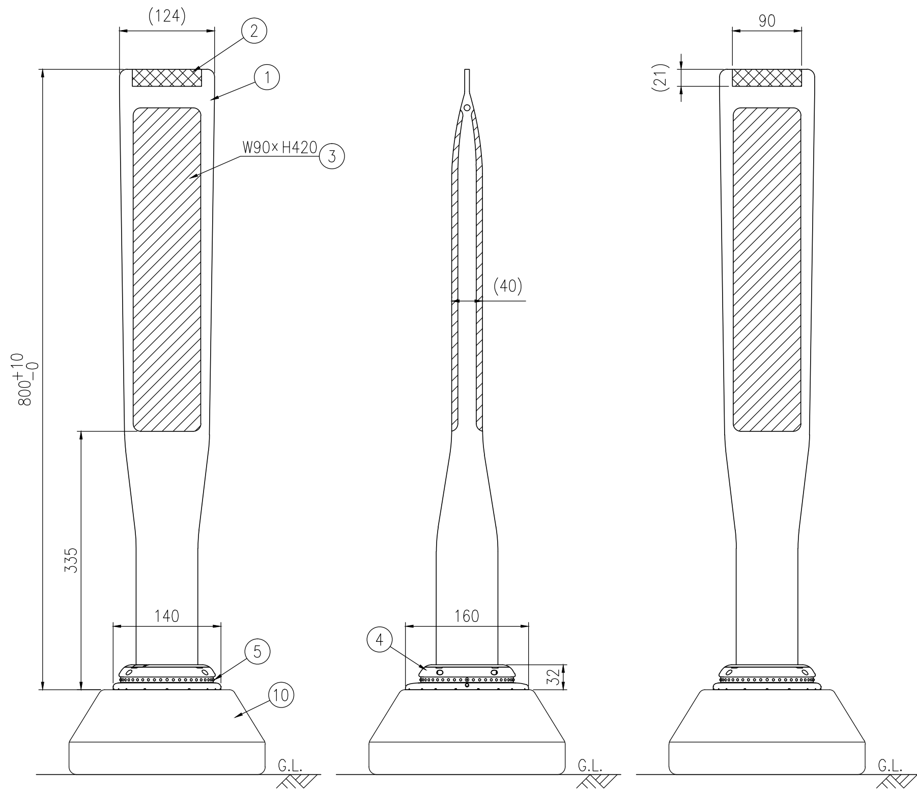
設置図 S=1/5
