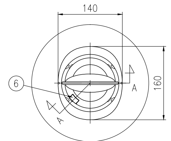
平面図 S=1/5
