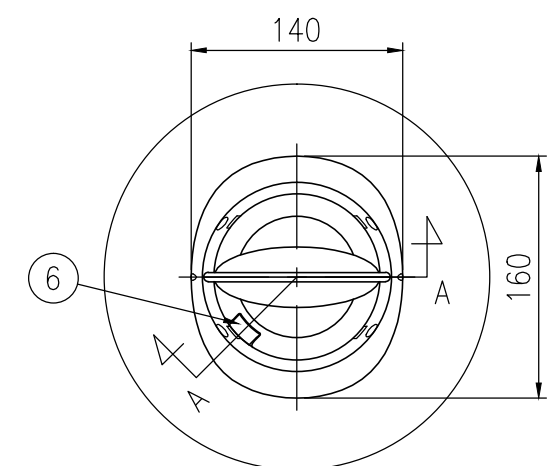
平面図 S=1/5
