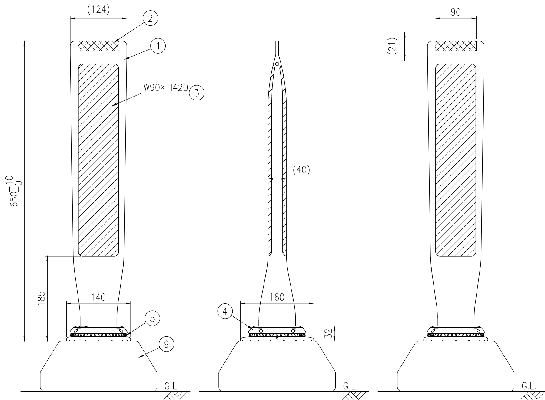
設置図 S=1/5
