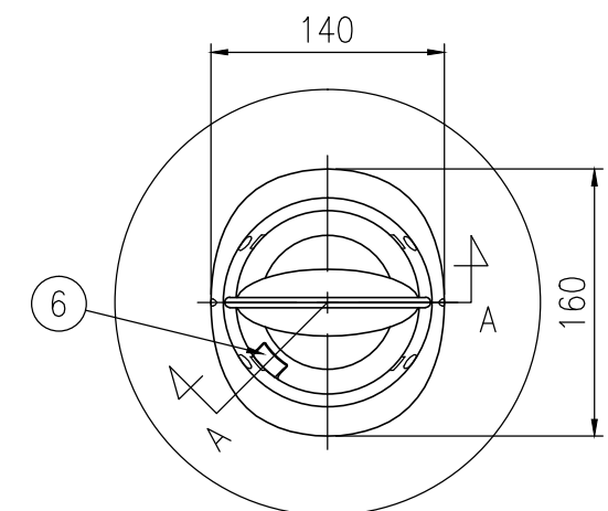
平面図 S=1/5
