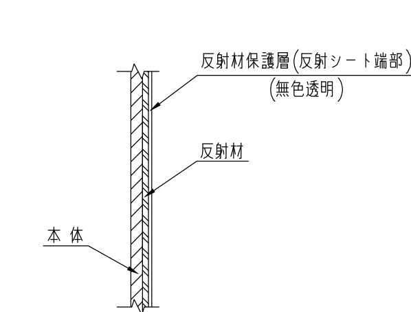
B部断面図
