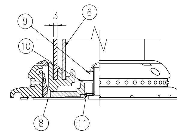
A-A半断面図 S=1/2
