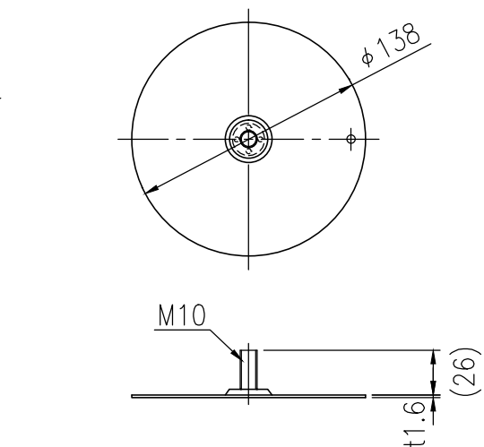
⑧ スチールスペーサー 詳細図 S=1/4
