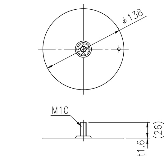
⑧ スチールスペーサー 詳細図 S=1/4
