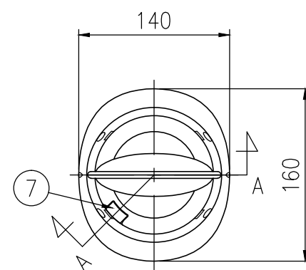
平面図 S=1/5
