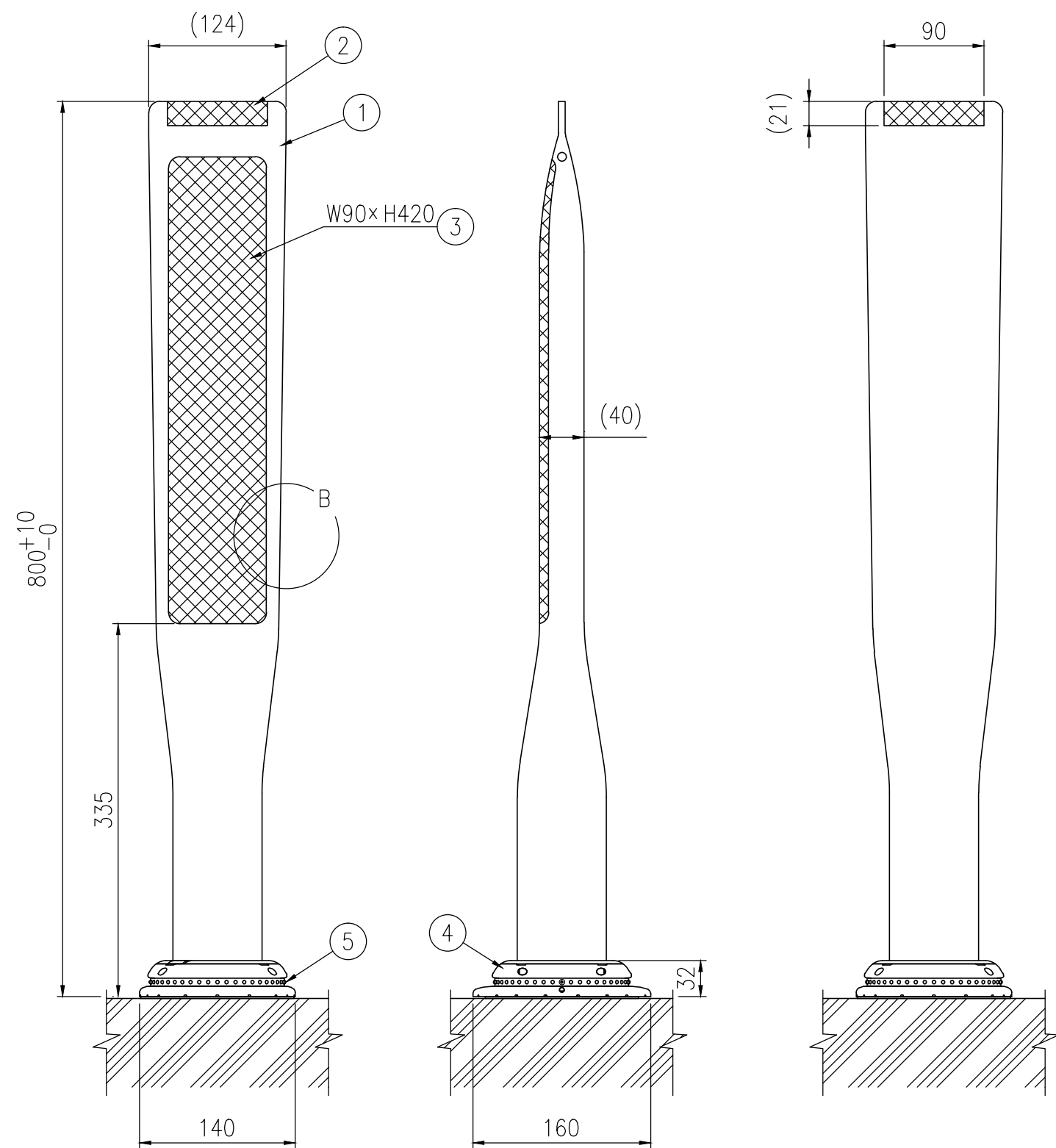
設置図 S=1/5
