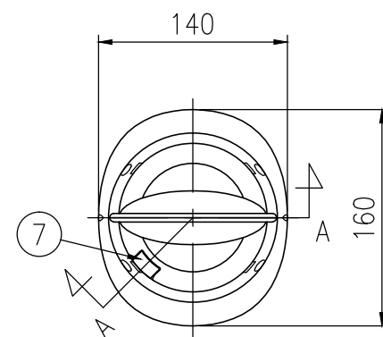
平面図 S=1/5
