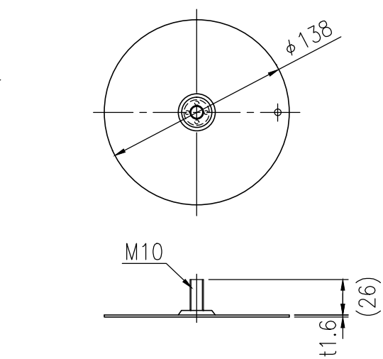
⑦ スチールスペーサー詳細図 S=1/4
