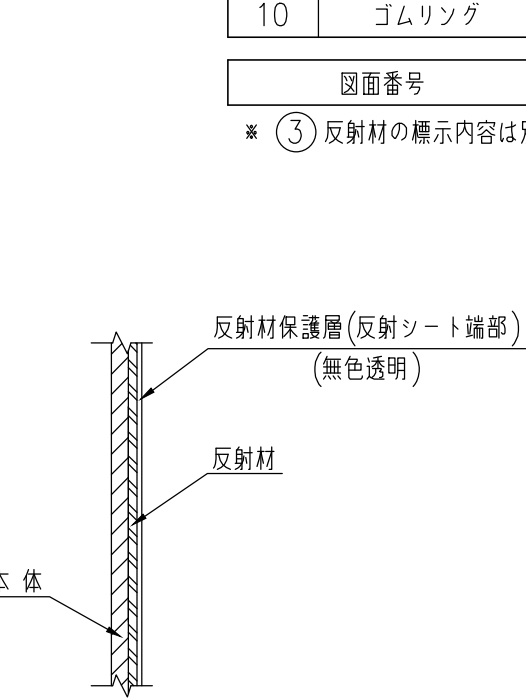
B部断面図
