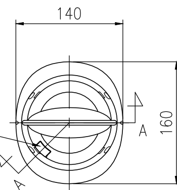
平面図 S=1/5
