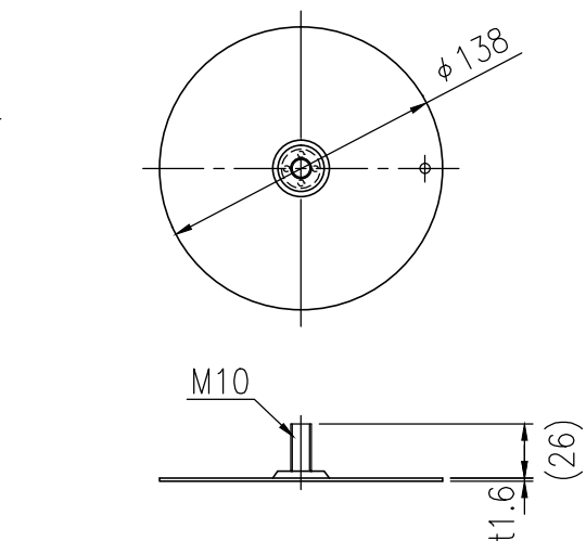
⑦ スチールスペーサー 詳細図 S=1/4
