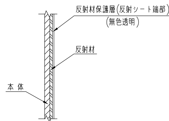
B部断面図
